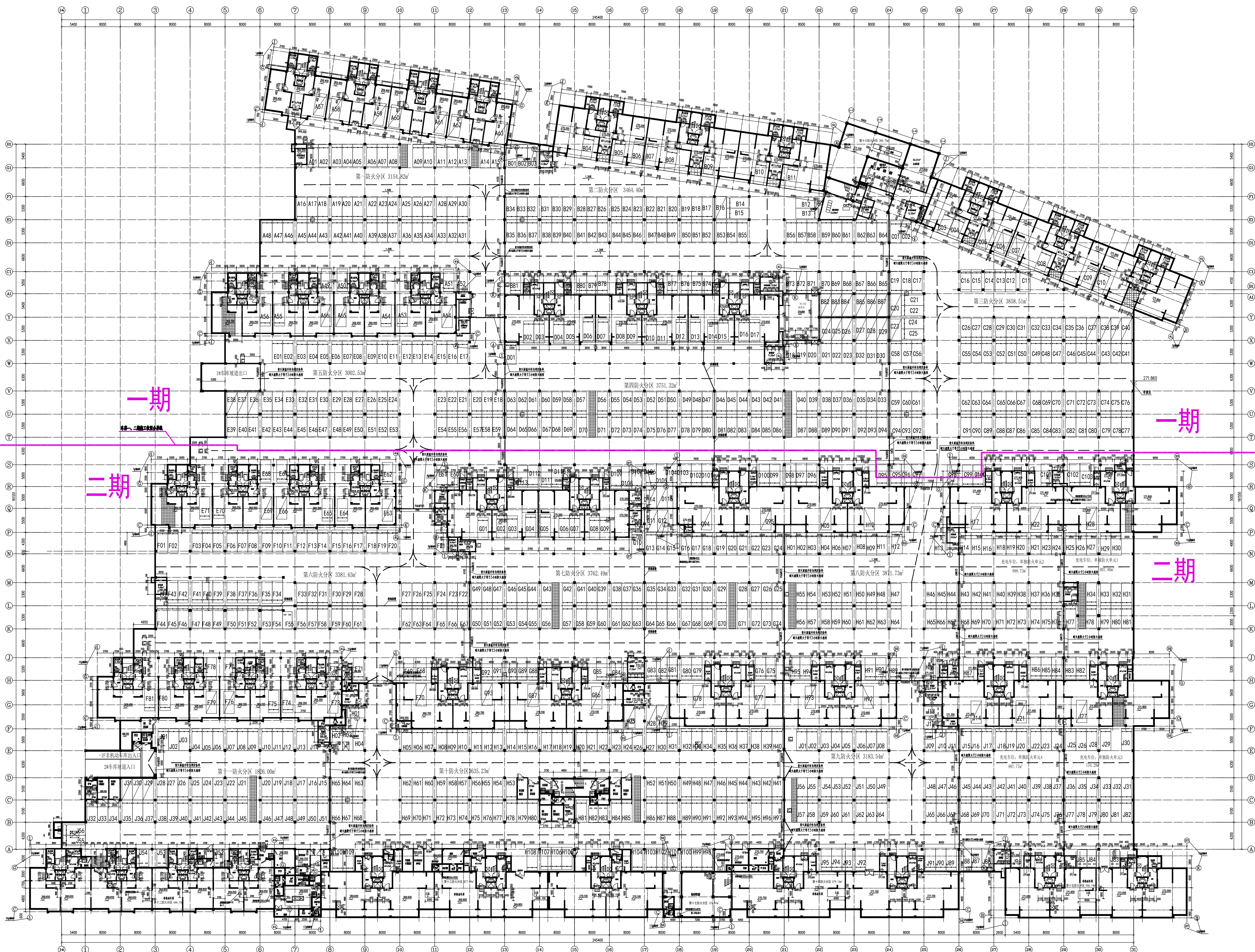
一、二期地下车库施工位置分界示意图 1:300
